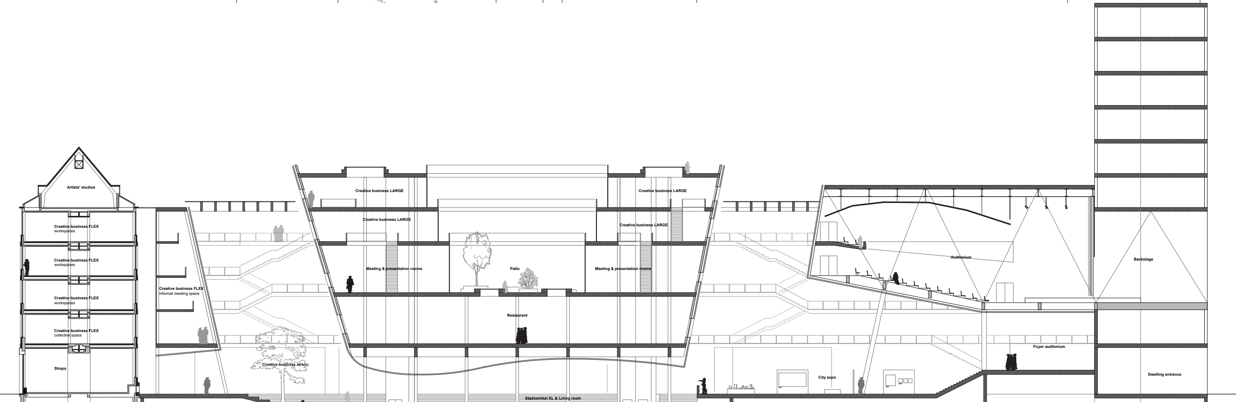
Long section B-B' 1:400
