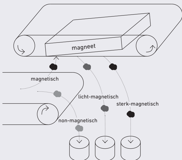
Figuur 7. Schematische tekening van de continue magnetische scheiding.
