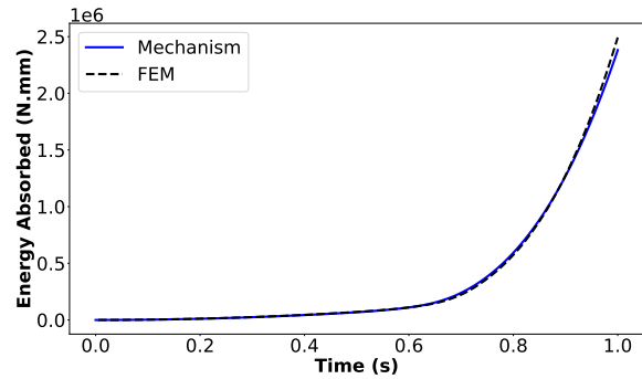
(d) Energy absorption: Rectangular simply supported
