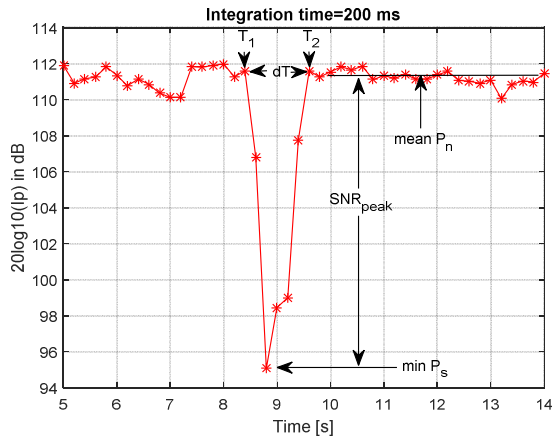
Figure 2. GPS Shadow Parameters
