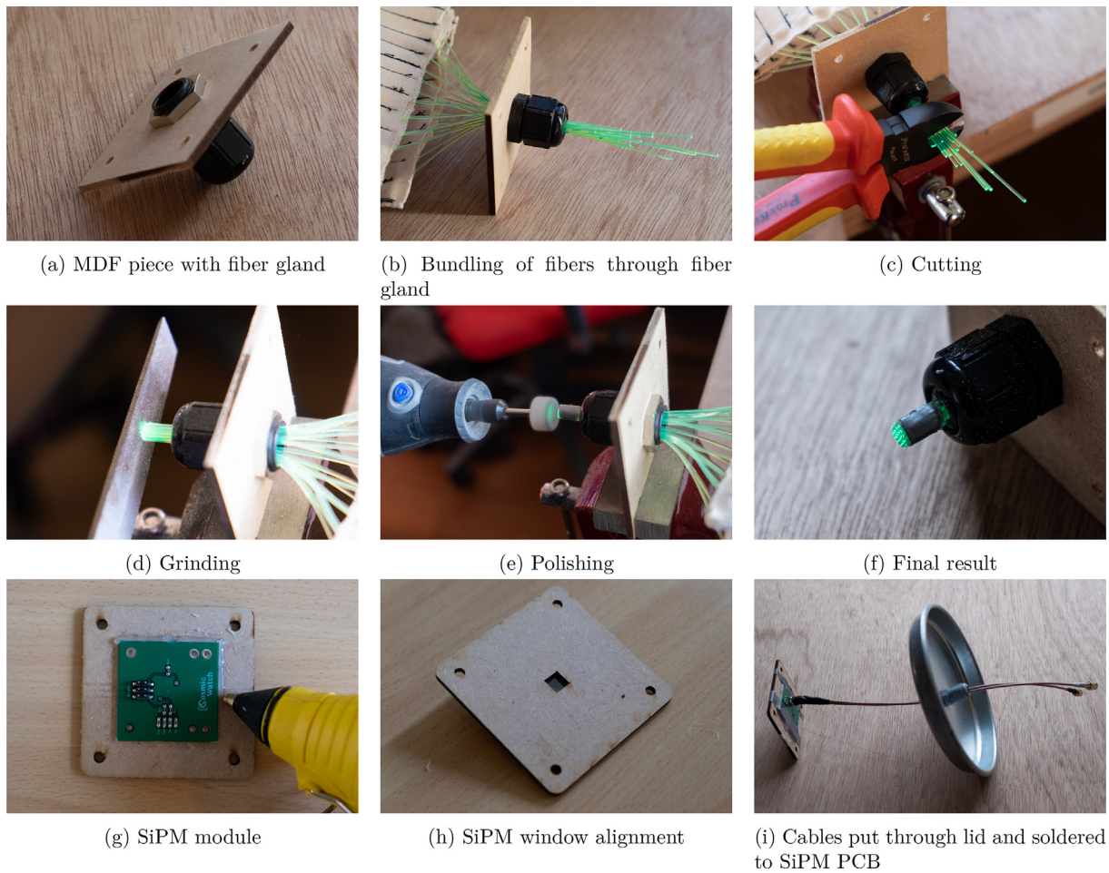
Fig. 5. SiPM Module.
