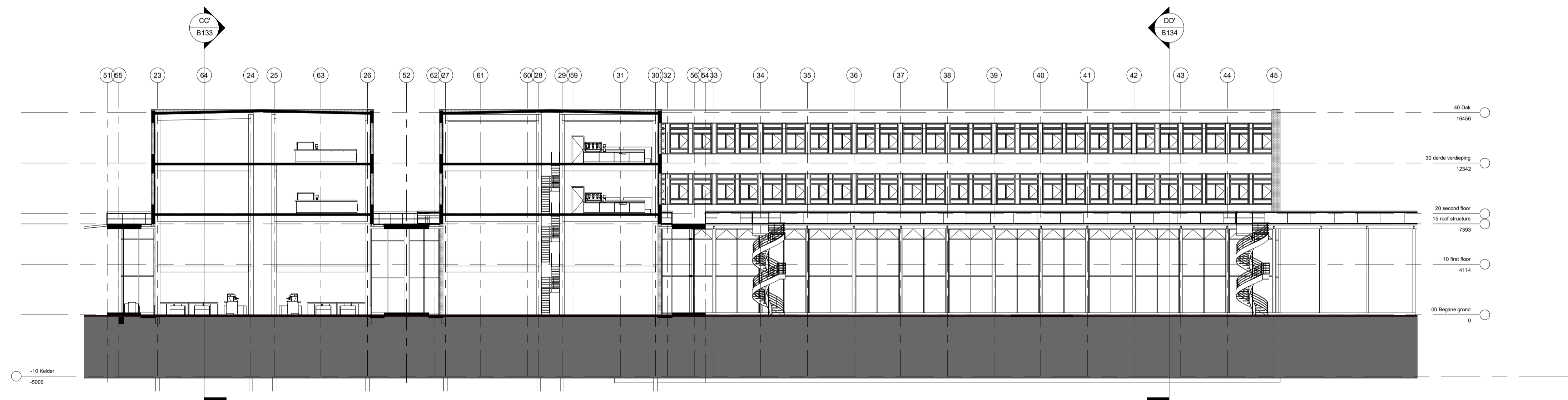
2 20 BB' 1/200 1 : 200
