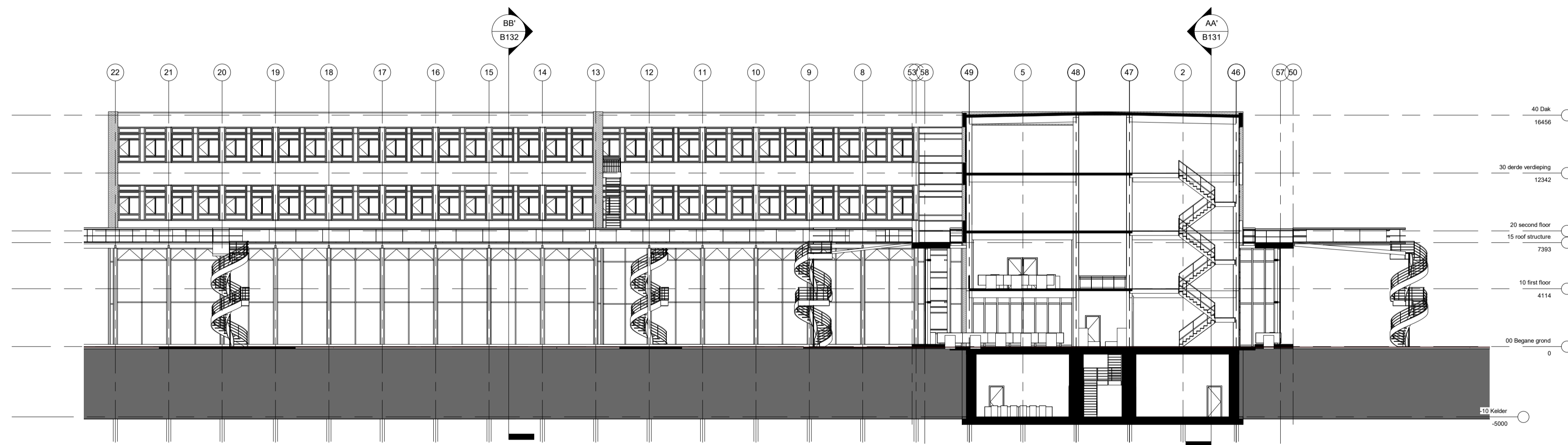
2 40 DD' 1/200 1 : 200
