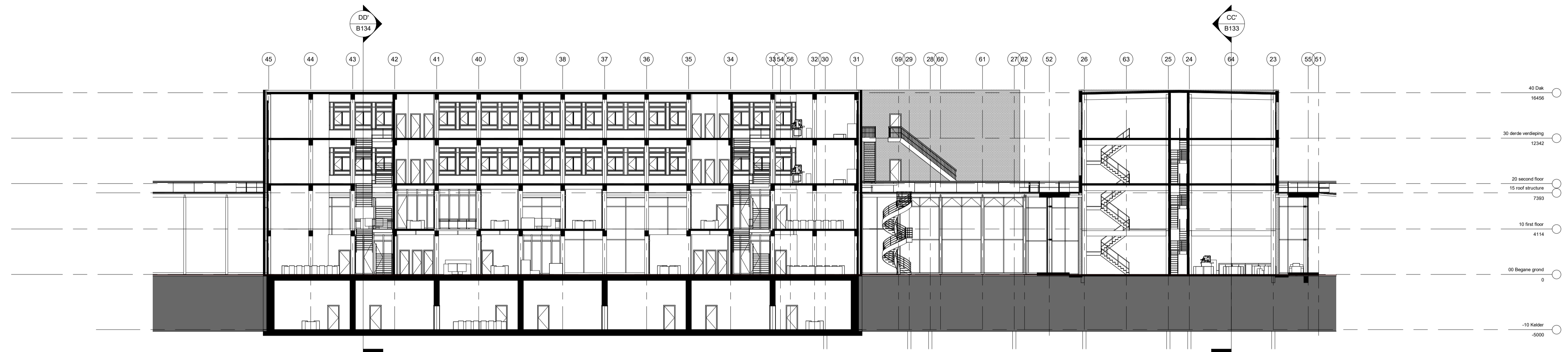
1 10 AA' 1/200 1 : 200
