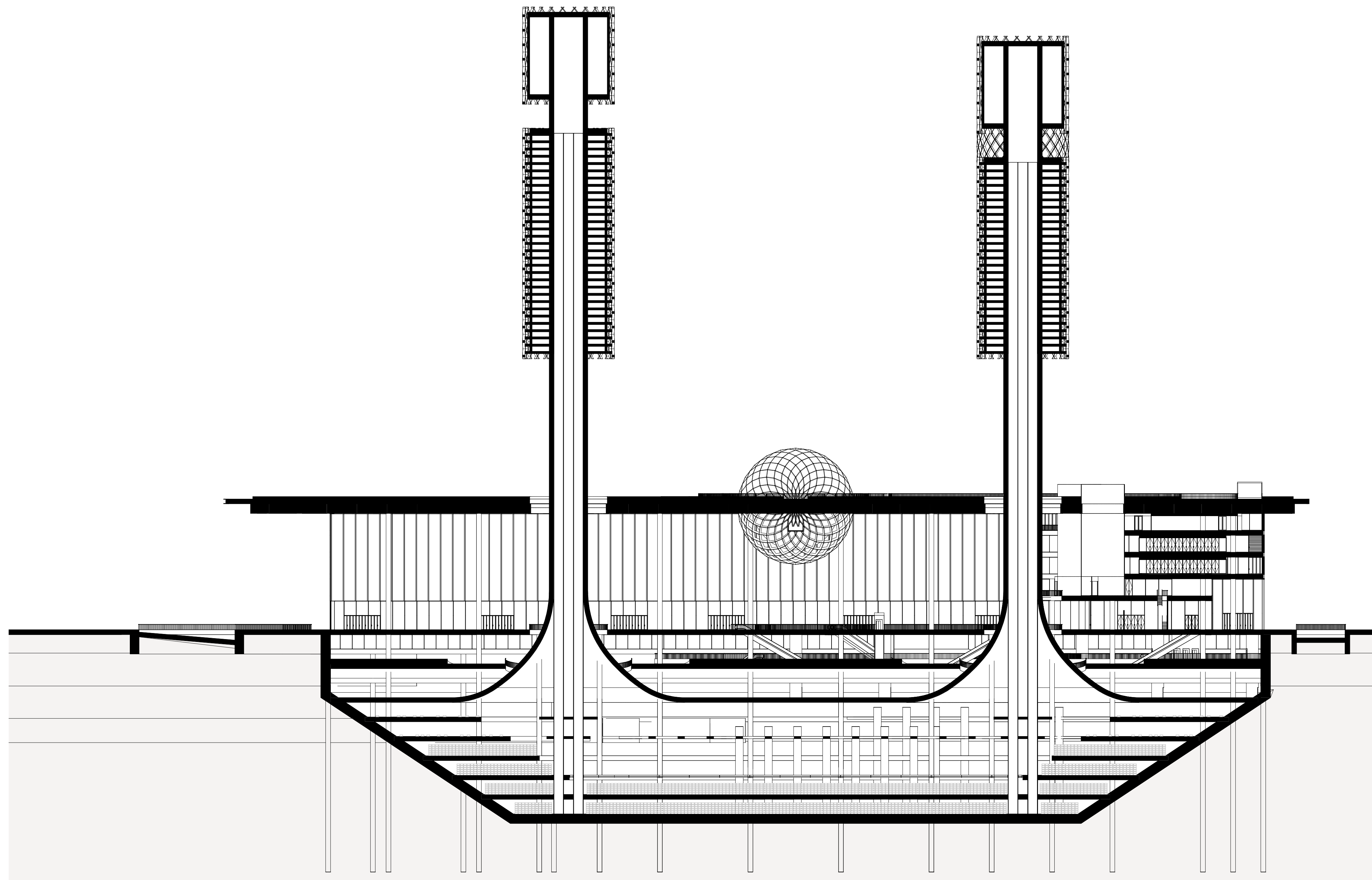
Longitudinal section | 1:500
