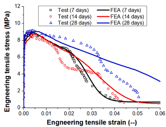
(b) UHPCFRC
