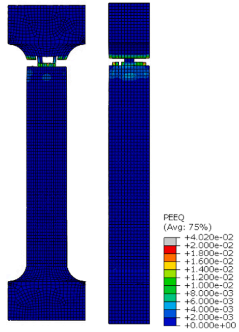
(b) UHPCFRC at 7 day (Scale=1.0)
