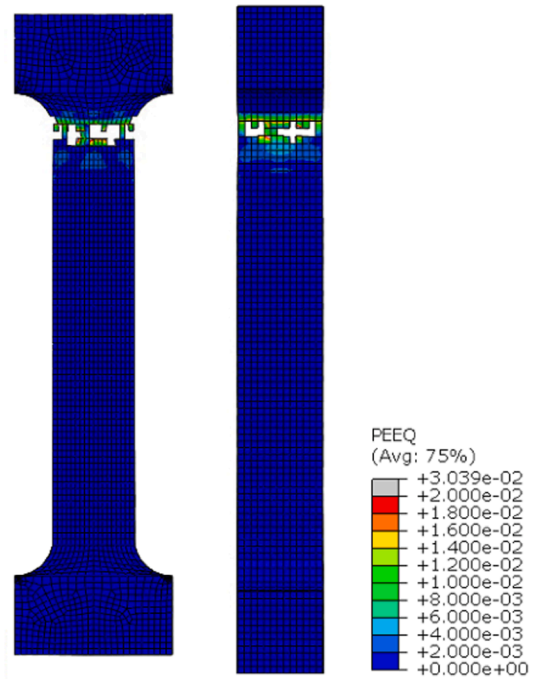
(d) UHPCFRC at 28 day (Scale=1.0)
