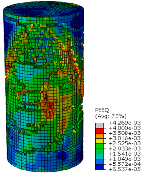
(d) UHPC (28 days) (Scale=0.1)
