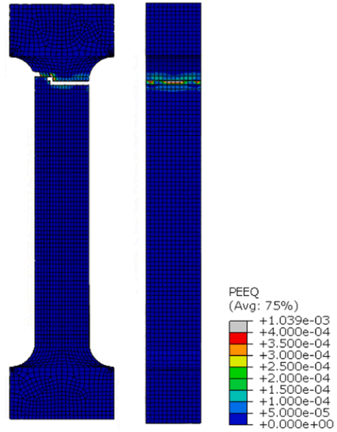
(d) UHPC (28 days) (Scale=1)
