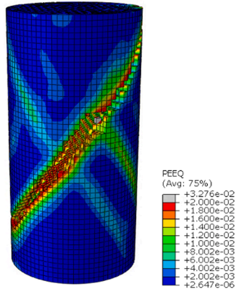
(d) UHPCFRC at 28 day (Scale=0.1)
