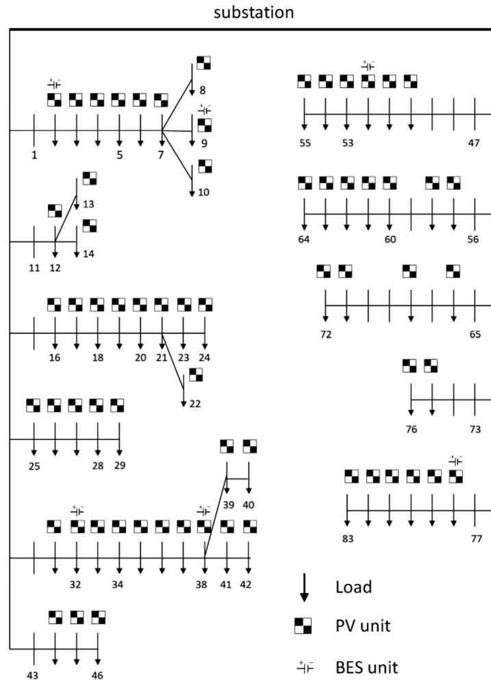
Fig. 9. Case C configuration. The sizes of the BES units (in kWh) are equal to: 300 (bus 2), 500 (bus 9), 300 (bus 32), 600 (bus 38), 500 (bus 52) 300 (bus 78).
