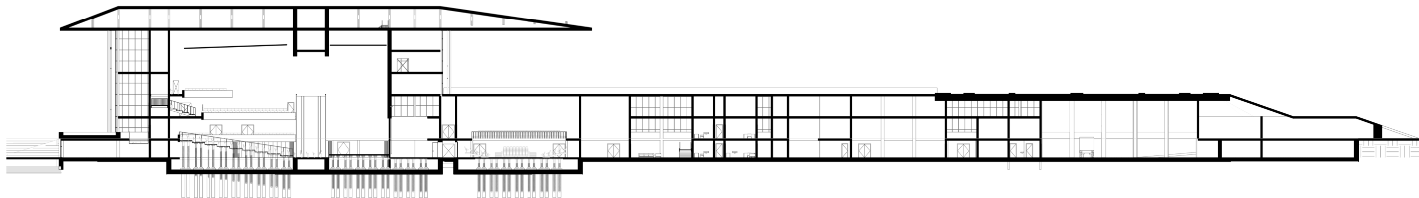
1 Doorsnede W-O 1 : 300
