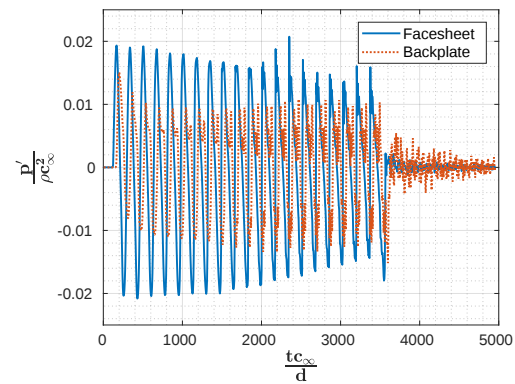
(d) SPL = 160 dB
