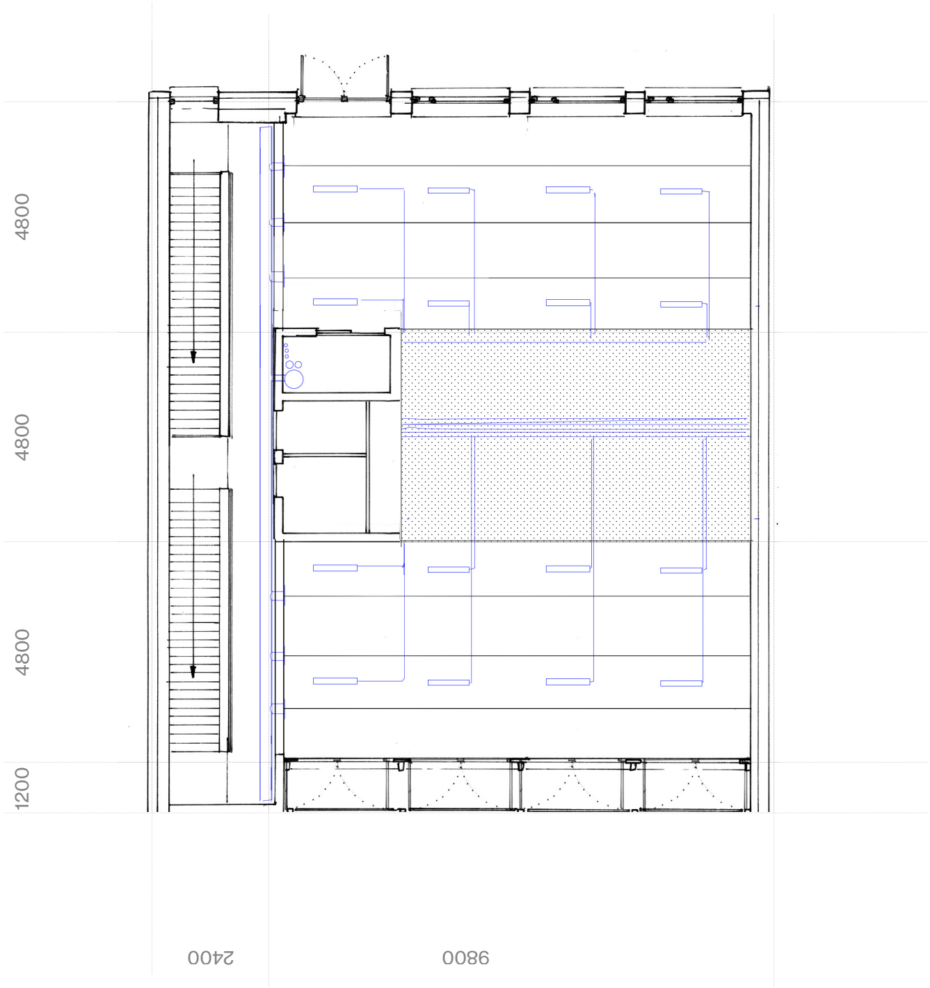
Plafond werkruimte
