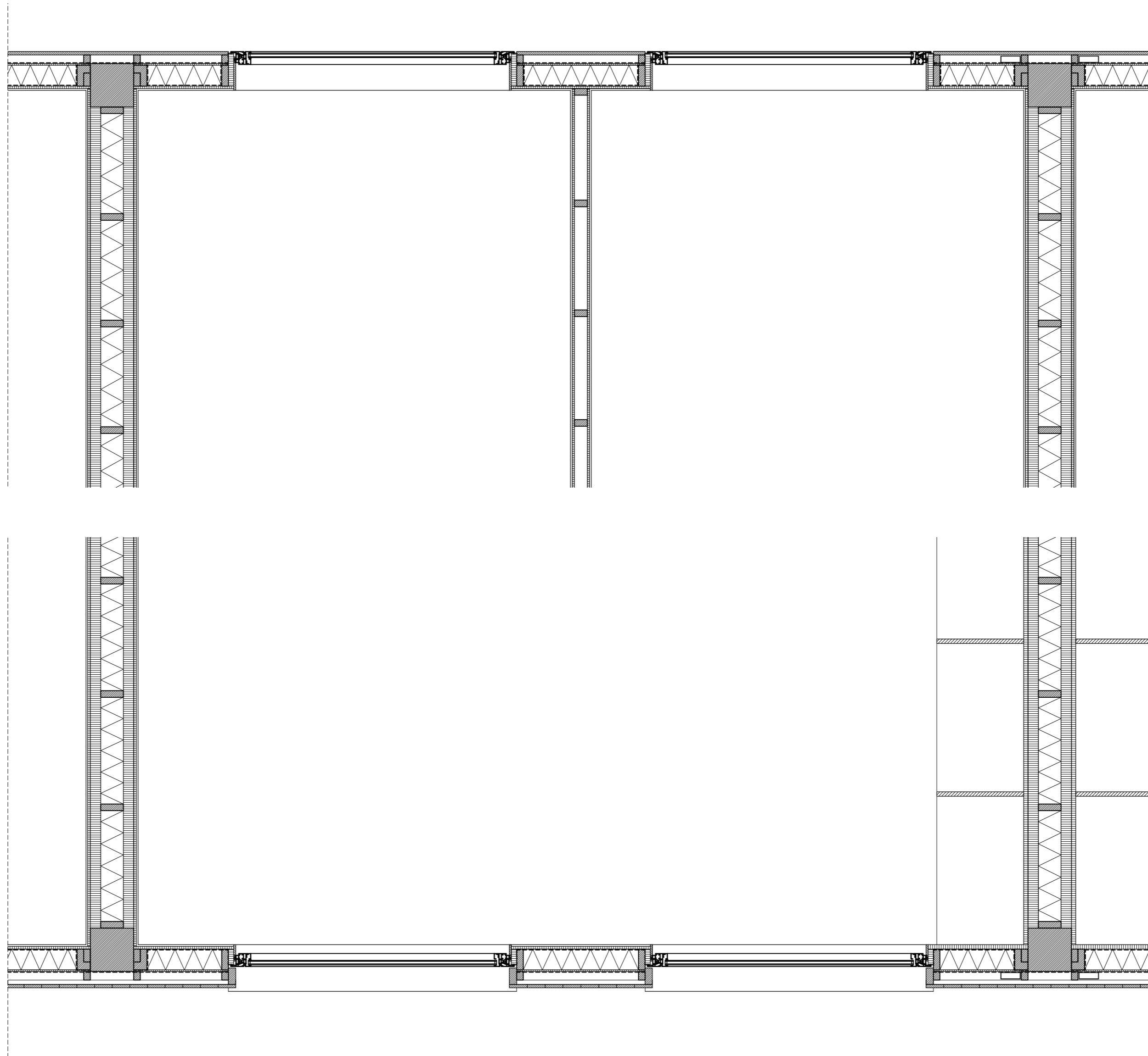
DOORSNEDE HORIZONTAAL +1 1:20
