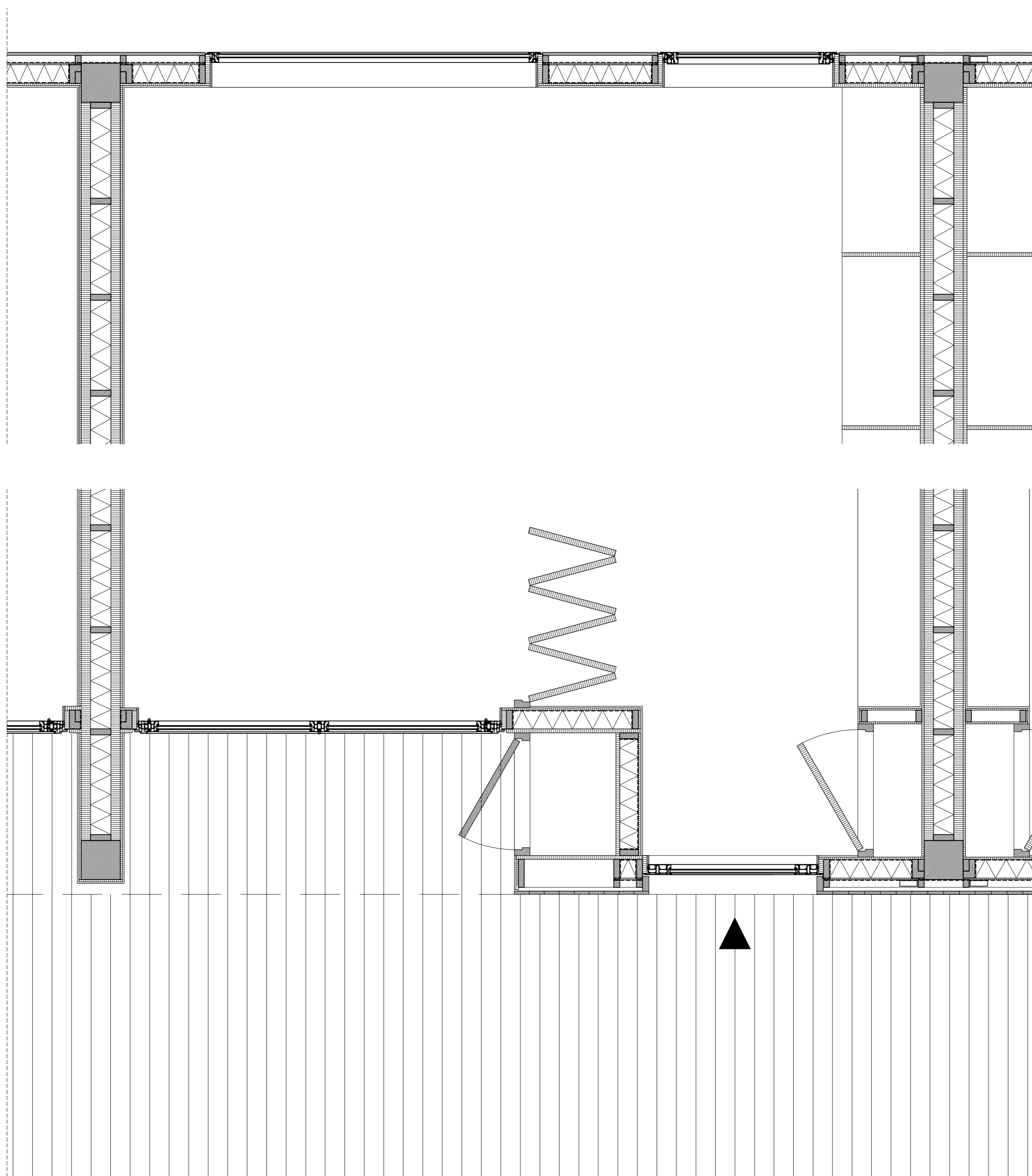
DOORSNEDE HORIZONTAAL BG 1:20
