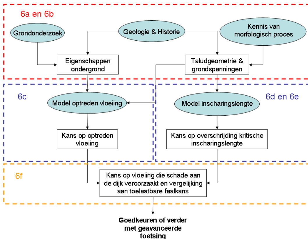
Figuur 6.1 Stappen om te komen tot de kans op een zettingsvloeiing die leidt tot schade aan de dijk, ten behoeve van de gedetailleerde toets
