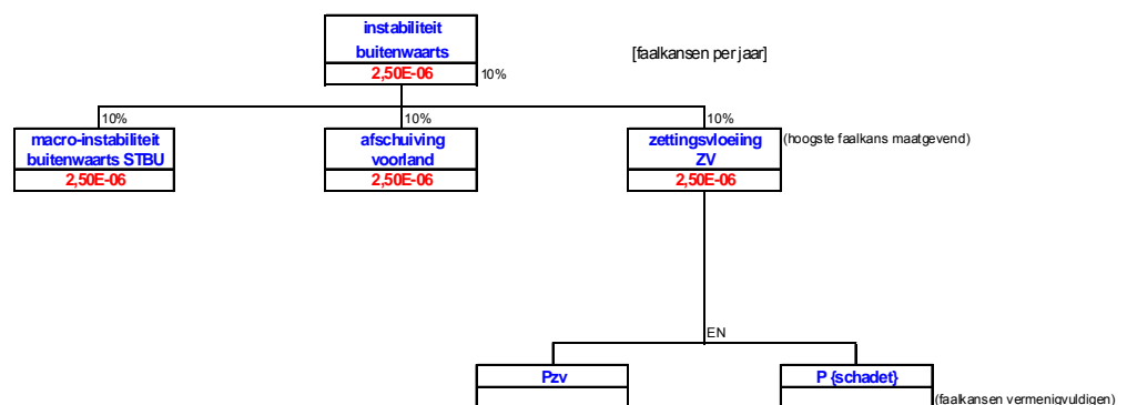
deelfoutenboom B dijkkring stabiliteit buitenwaarts
