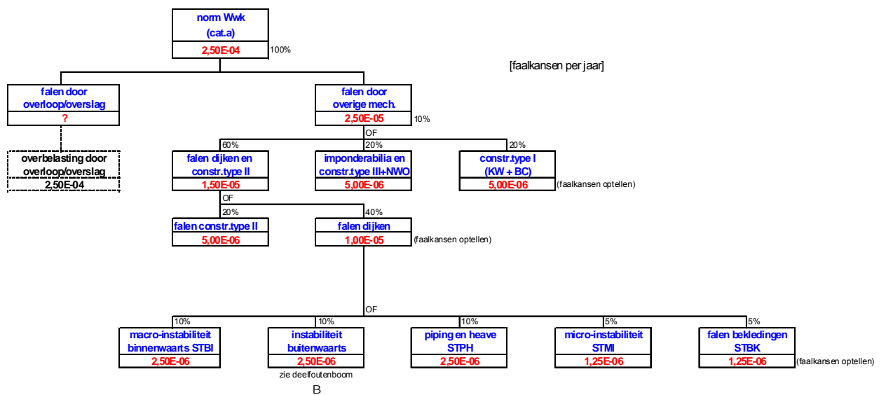
foutenboom A dijkkring
