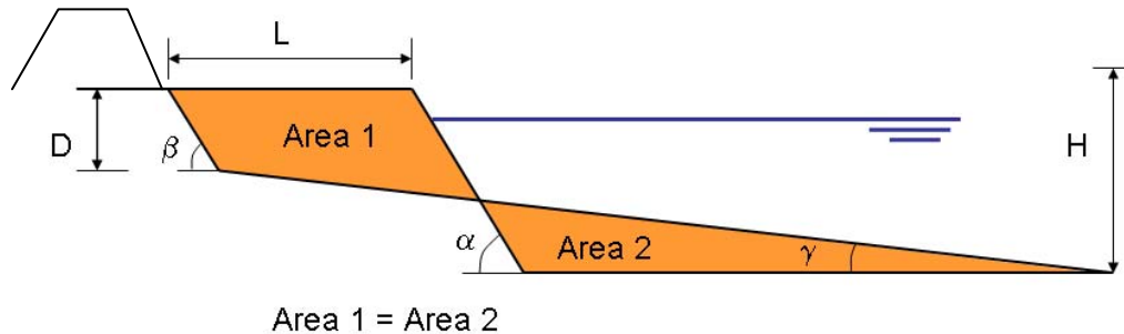
Figuur 6.2 Inscharingslengte na zettingsvloeiing [Silvis en De Groot 1995]
