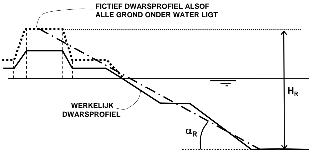
Figuur 5.1 Fictief onderwater dwarsprofiel; definitie van rekentaludhoogte H_R en rekentaludhelling \alpha_R
