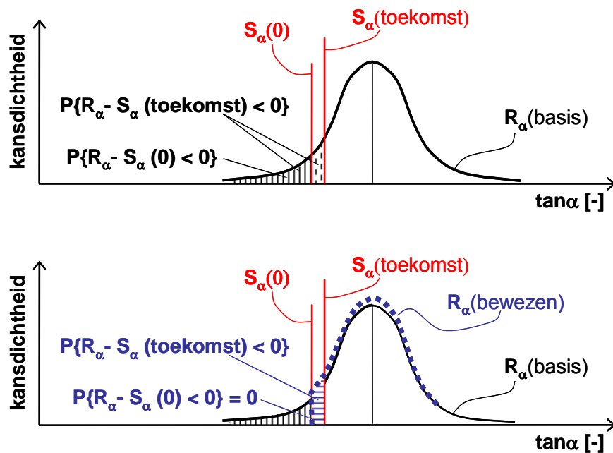
Figuur 6.3 Vertaling van kansdichtheid met medenemen van bewezen sterkte
