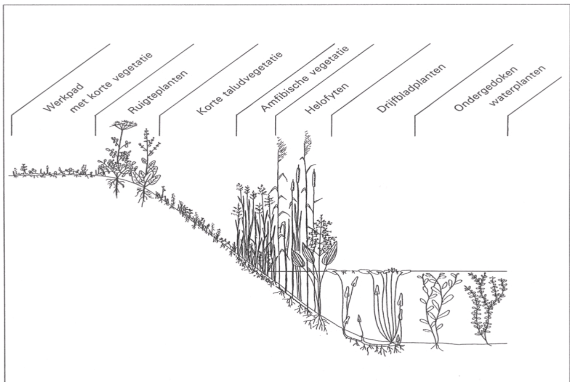
figuur 1 Zoneringschema; een houtzone kan in de plaats van een of méér droge zones liggen
