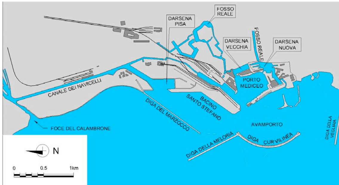
Figure 8. 1908 Port Plan (Eng. L. Cozza).
